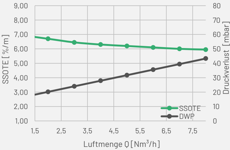
SSOTE und Druckverlust für HD270 F053A
