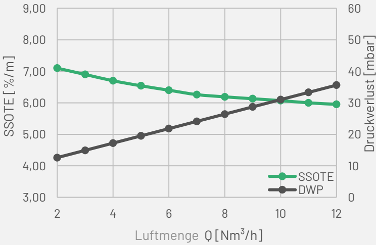
SSOTE und Druckverlust für HD300+ F053A
